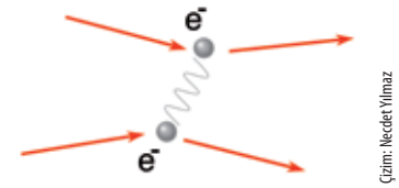
Fonon aracılığıyla bir arada tutulan elektron çifti (Cooper çifti)
